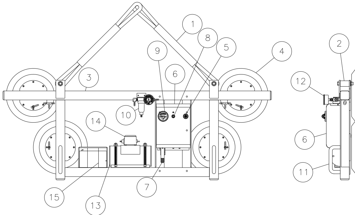
Abbildung des Hebegerätes VL411LDC (Standard-Modell)
