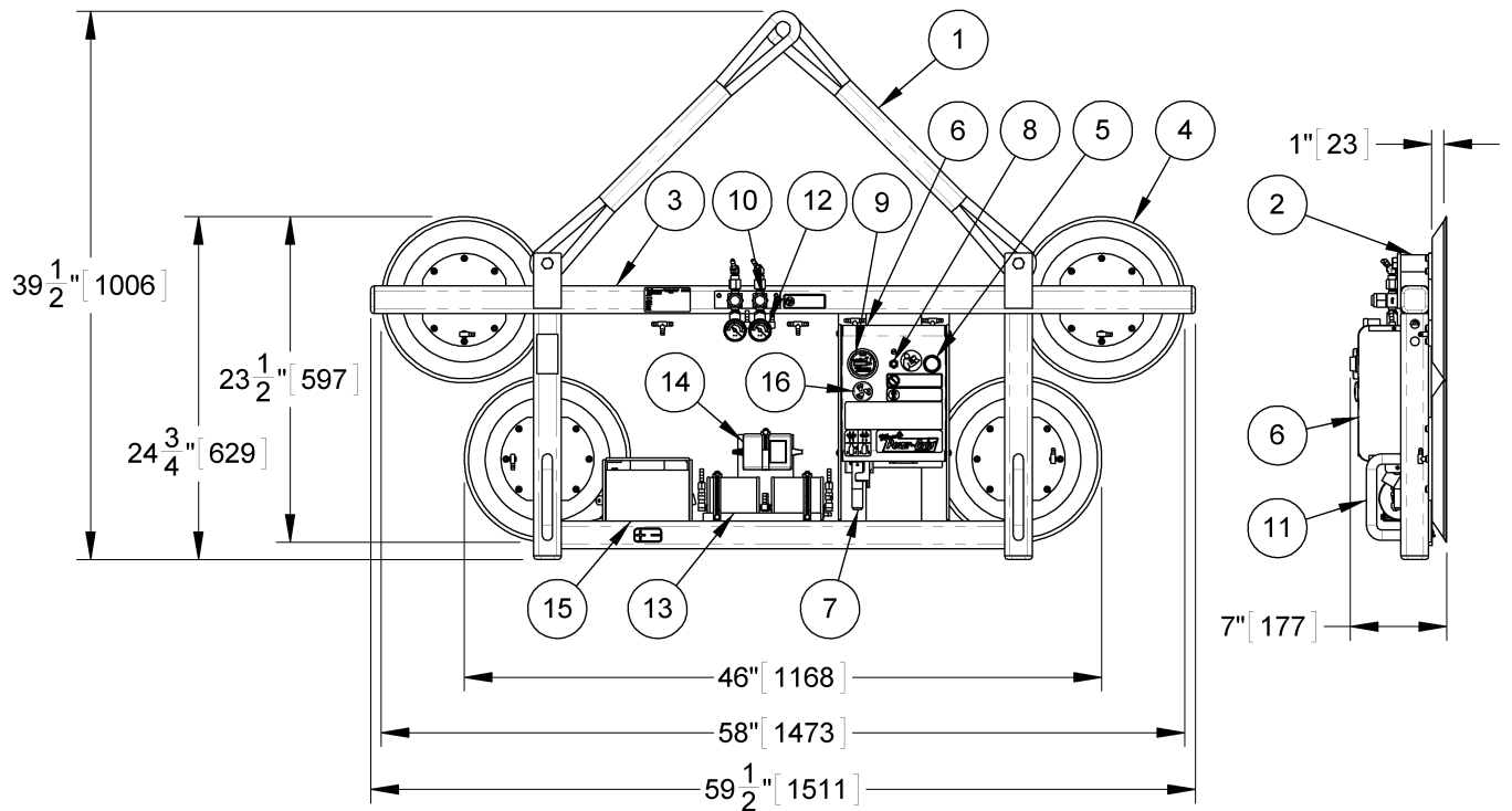
Schéma du modèle standard VL411LDC avec double circuit de vide facultatif.
